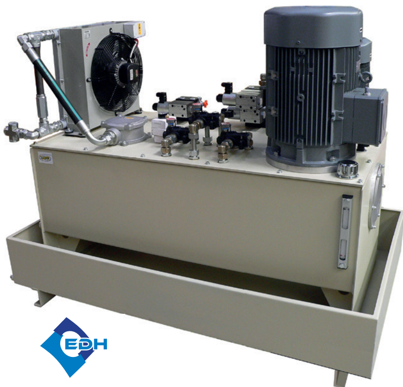
Réservoirs EDH sur-mesure
